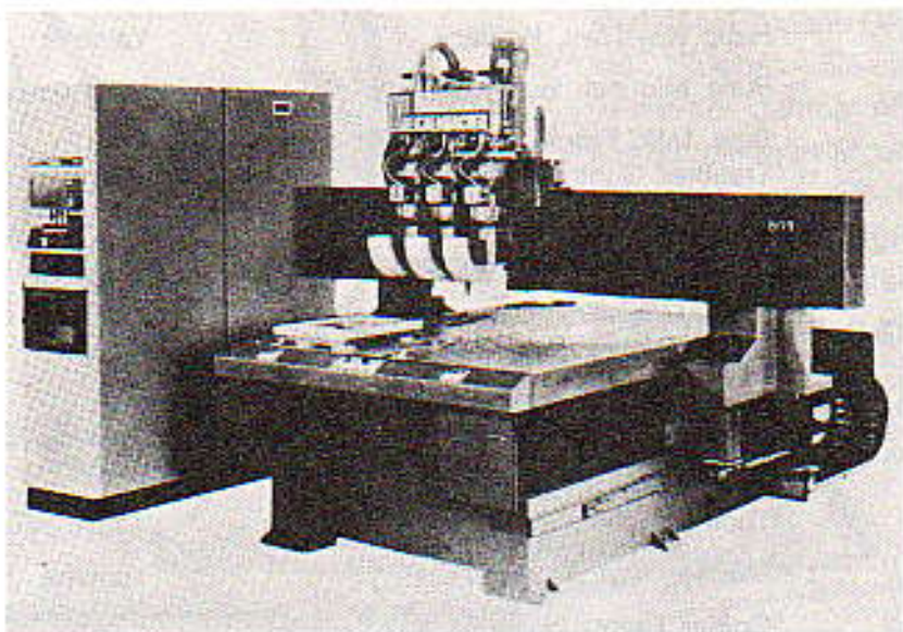
CNC-gesteuerte Fräsmaschine
