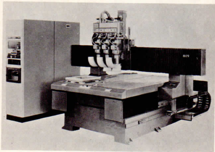
CNC-gesteuerte Fräsmaschine
